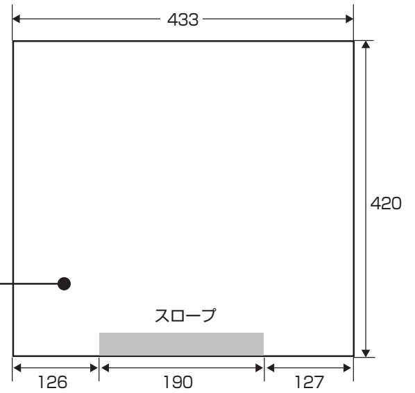
床面 平面図
