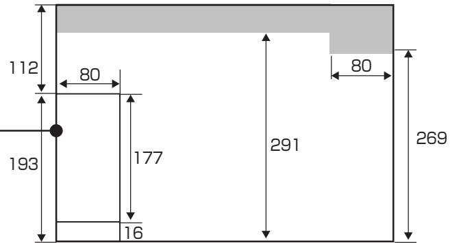
正面 平面図
